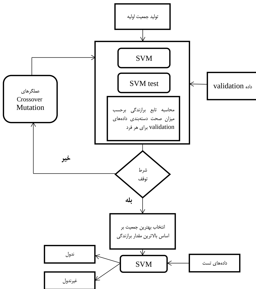
شکل ۵: الگوریتم پیشنهادی
