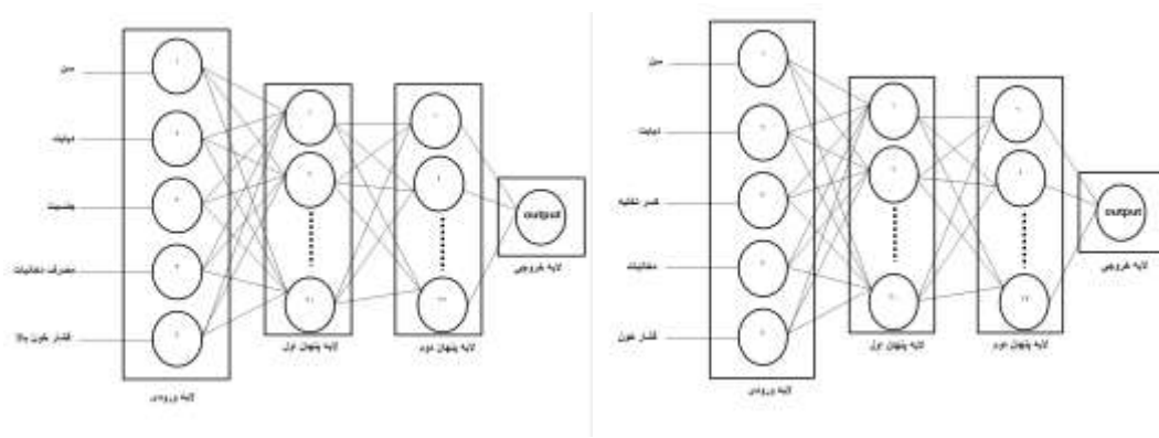
شکل ۲-۲ طراحی شبکه عصبی N2 با ورودی‌های سن- دیابت- کسر تخلیه- مصرف دخانیات- فشارخون
