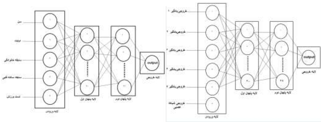
شکل ۲-۶ طراحی شبکه عصبی راهگامی با ورودی‌های شبکه عصبی N1 تا N6
