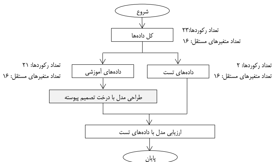
شکل ۱: مدل درخت تصمیم پیوسته پیشنهادی
