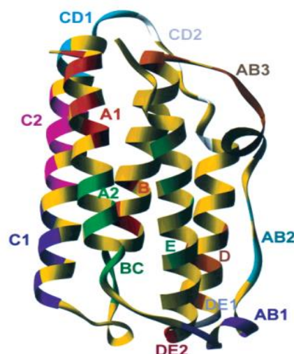
شکل ۱: ساختار سه بعدی اینترفرون بتای انسانی
