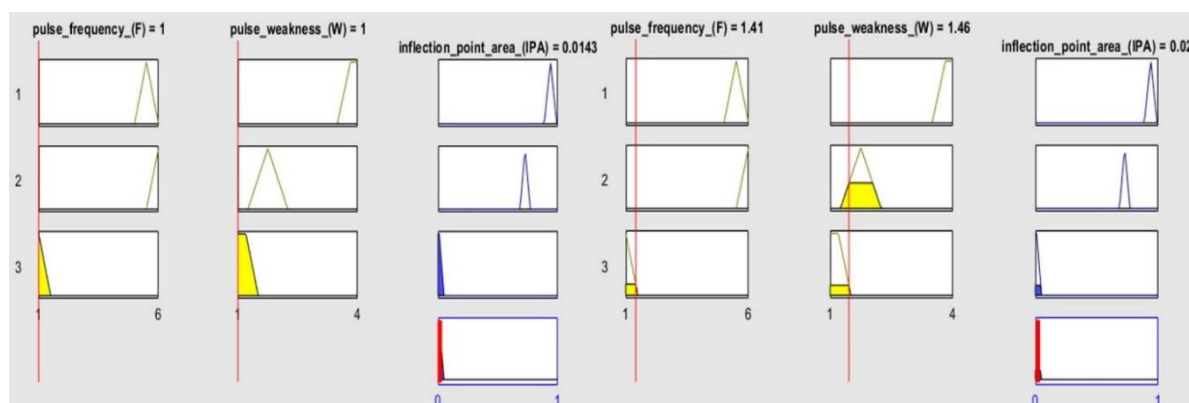
شکل ۸: الف. حداکثر مقدار خروجی 0.2/0 بر اساس مقادیر ورودی قانون سوم شکل ۸: ب. حداقل مقدار خروجی 0.143/0 بر اساس مقادیر ورودی قانون سوم
