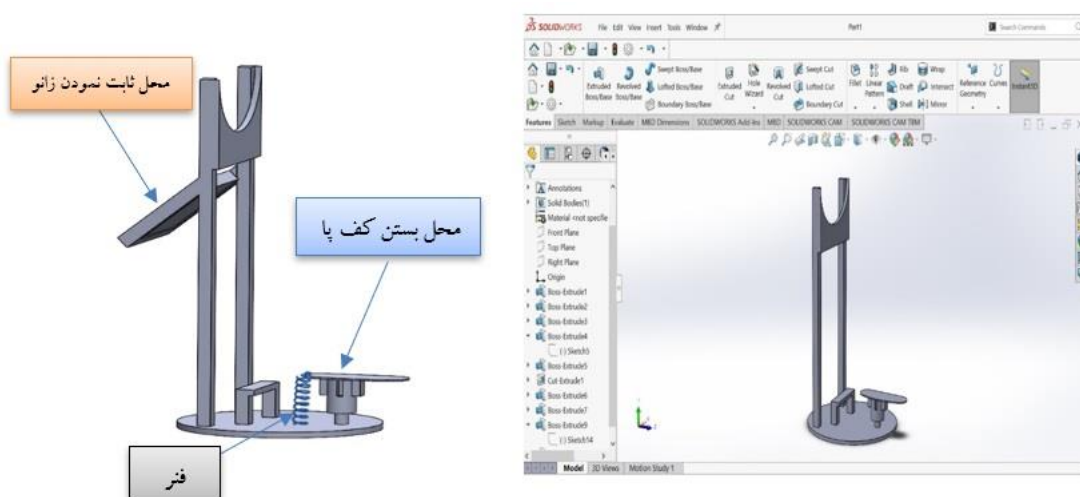
شکل ۲: مدل طراحی شده در نرم افزار سالیدورکس
