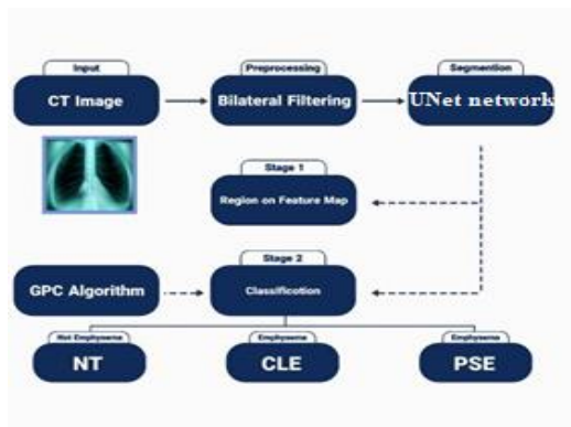
شکل ۶: مراحل روش پیشنهادی
