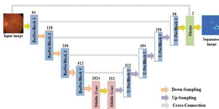
شکل ۳: ساختار شبکه U-Net
