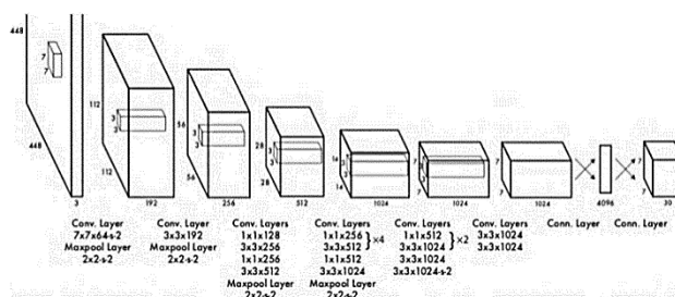
شکل ۳: ساختار شبکه YOLO
