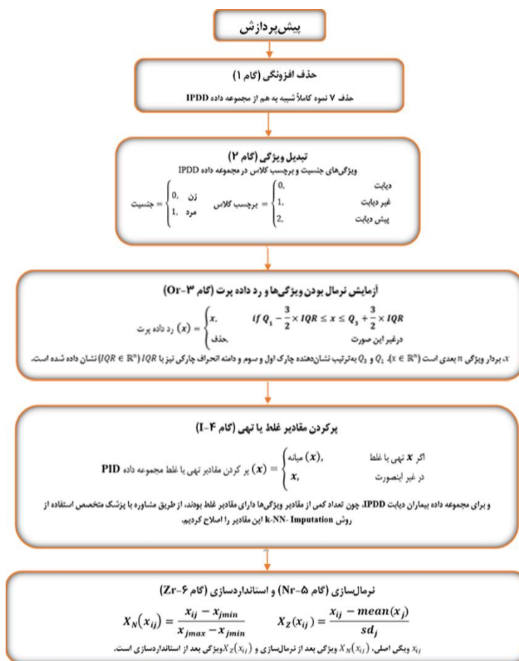
شکل ۲: گام‌های پیش‌پردازش
