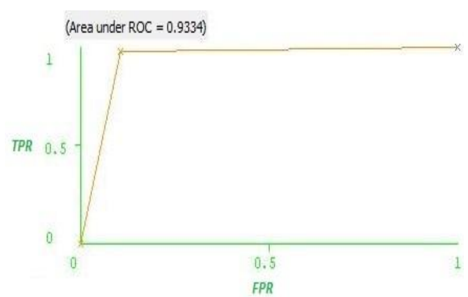
SVM
